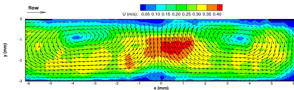
Рис. 8. Двух-вихревое течение в горизонтальном слое этанола, газ - воздух, U_{\text{gas}}=13.8 см/с, H=3 мм, T=20^\circ\text{C} , [18,19].
