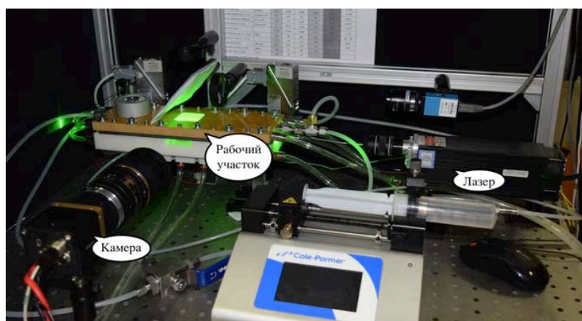
Рис. 7. Экспериментальный стенд для исследования испарения с локальной поверхности горизонтального слоя жидкости, обдуваемой потоком инертного газа, [7,52].
