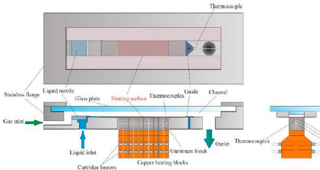
Рис. 41. Дизайн рабочего участка, [6,31].
