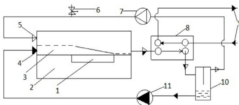
Рис. 36. Концепция системы охлаждения электронного оборудования с использованием чистого пара и парогазовой смеси: 1 –электронный компонент; 2 – подложка; 3 – испаряющаяся плёнка жидкости; 4 – вход жидкости в канал; 5 – вход парогазовой смеси в канал; 6 – клапан для сброса и регулировки концентрации неконденсируемого газа; 7 – компрессор; 8 – пластинчатый теплообменник (конденсатор пара); 9 – система охлаждения конденсатора; 10 – сепаратор, совмещенный с баком-накопителем для жидкости и газовой фазы; 11- жидкостный насос, [112].
