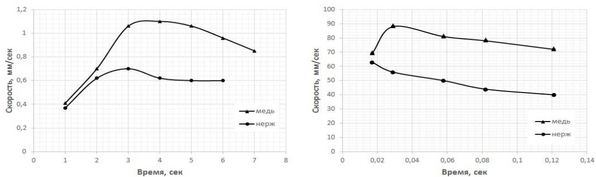
Рис. 21. Скорость распространения линии контакта для пленки воды на поверхностях с различной смачиваемостью: h=0,4 мм, q=27 Вт/см 2 , слева - \theta_a=27\pm 3^\circ , справа - \theta_a=74\pm 5^\circ , [37,46].
