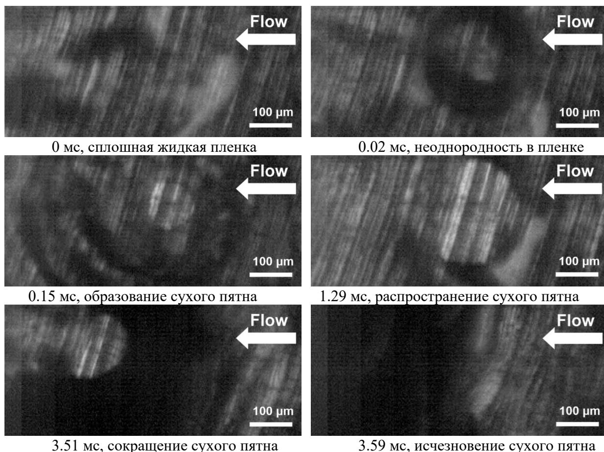
Рис. 47. Динамика сухого пятна. Число Рейнольдса жидкости Re_l=40 , приведенная скорость газа U_{sg}=19,5 м/с, тепловой поток q=450 Вт/см 2 , температура поверхности нагревателя T_w=130^\circ\text{C} , поток направлен справа налево. Частота съемки — 100 000 кадров в секунду, [103].
