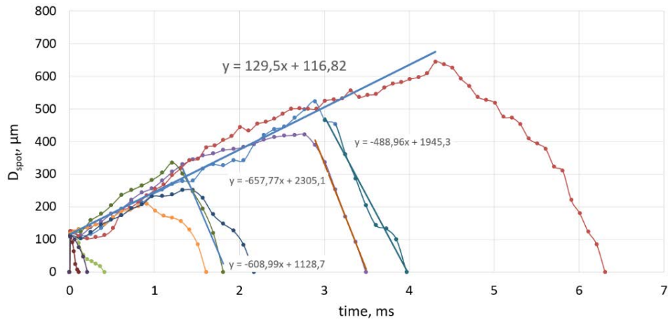
Рис. 50. Зависимость среднего диаметра сухого пятна от времени. Те же параметры эксперимента, что указаны на Рис. 9, [103].
