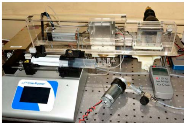
Рис. 10. Фотография экспериментального стенда для исследований по динамике и теплообмену в области линии контакта газ – жидкость – твердое тело, [29,30].
