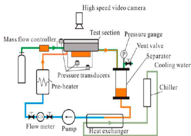
Рис. 40. Схема экспериментального стенда, созданного иностранным партнером, [6,31].
