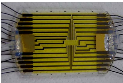
Рис. 13. Фотография нагревательного элемента на основе сапфира с прозрачным нагревателем ITO изготовленного иностранным партнером.
