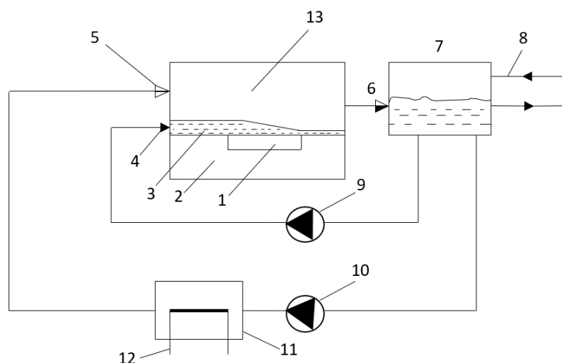
Рис. 35. Концепция системы охлаждения электронного оборудования с использованием чистого пара: 1 –электронный компонент; 2 – подложка; 3 –испаряющаяся плёнка жидкости; 4 – вход жидкости в канал; 5 – вход пара в канал; 6 – вход жидкости и пара в конденсатор; 7 – конденсатор пара и резервуар для жидкости; 8 – система охлаждения конденсатора; 9 –насос для подачи жидкости в канал; 10 – насос для подачи жидкости в парогенератор; 11- парогенератор и резервуар для пара; 12- электрический подогреватель; 13 – мини или микро-канал, [111].
