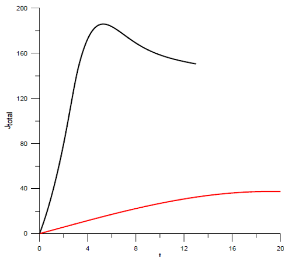
Рис. 5. Безразмерная скорость суммарного испарения с границы раздела газ/пар – жидкость в зависимости от безразмерного времени (реальное время развития процесса 4 с): черная линия - газ азот; красная линия - водяной пар, размер нагревателя 3 x 6 мм, высота канала H_C=300 мкм, T_0=30^\circ\text{C} , Re_l=2.5 , Re_g=4 , q=0.5 Вт/см 2 , [30].
