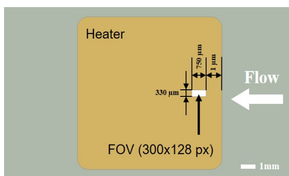
Рис. 46. Поле зрения камеры при съемке с частотой 100 000 кадров/секунду.
