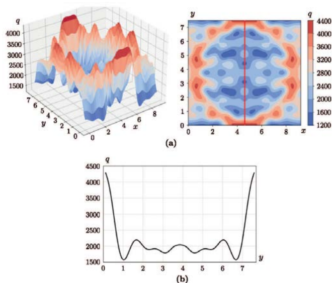
Рис. 9. Локальный тепловой поток, вычисленный методом тонкой фольги. плотность теплового потока существенно возрастает вблизи линии контакта газ–жидкость–твёрдое тело [1].
