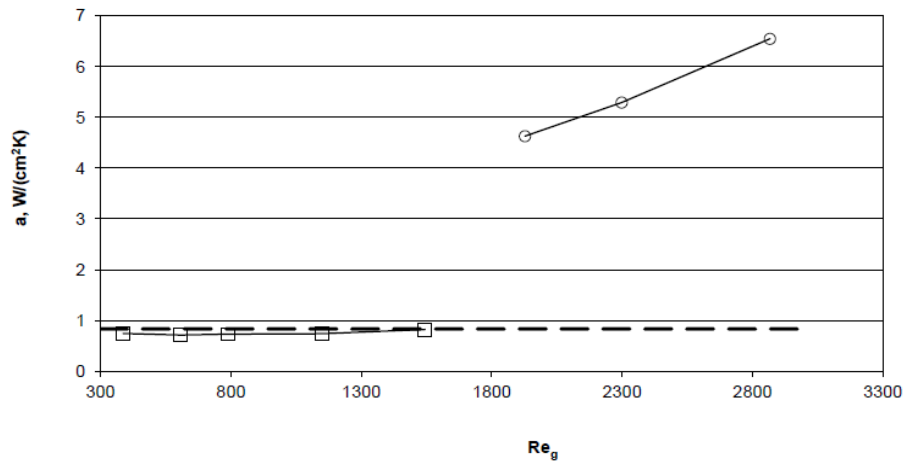
Рис. 28. Зависимость коэффициента теплоотдачи от числа Re газа. За характерную температуру жидкости при температуре стенки более 100\text{ }^{\circ}\text{C} принимается температура насыщения (круглые значки), а при температуре стенки менее 100\text{ }^{\circ}\text{C} принимается начальная температура пленки (квадратные значки). Пунктир - коэффициент теплоотдачи для стекающей пленки, [30].
