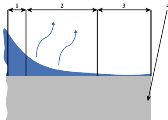
Рис.2 Схема переходной области (2) между макромасштабным мениском (1) и адсорбированной пленкой жидкости (3). (4) – подложка.
