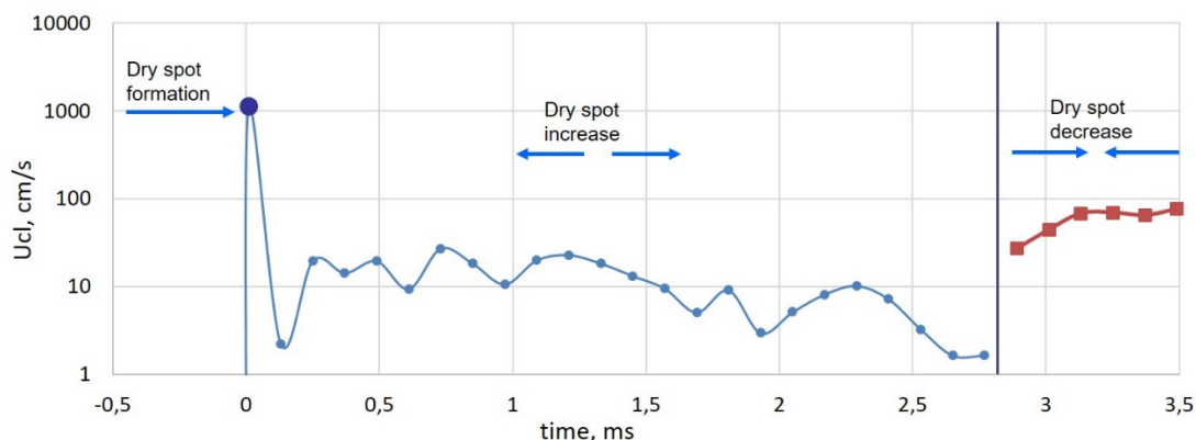
Рис. 49. Скорость линии контакта на этапах формирования, распространения и схлопывания. Все параметры потока такие же, как на Рис. 9.
