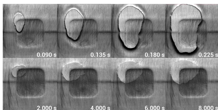
Рис. 20. Влияние смачиваемости подложки на скорость распространения сухого пятна в пленке воды толщиной h=0,4 мм, q=27 Вт/см 2 (съемка 5000 кадров/сек): верхняя линия фото - \theta_a=74\pm 5^\circ ; нижняя линия фото - \theta_a=27\pm 3^\circ , [37,46].
