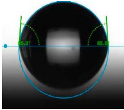
Рис. 16. Изучение динамической смачиваемости нагревательного элемента (поверхность сапфира), [31].
