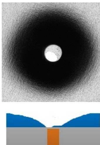
Рис. 24. Формирование плоского остаточного слоя сверхтонкой пленки жидкости перед разрывом слоя макропленки (шлирен изображение и схема): этанол, h = 700 мкм, q = 95 Вт/см 2 , \Theta_a = 8 \pm 1^\circ , полированная поверхность, [43,48].
