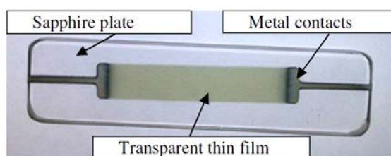
Рис. 15. Фотография сапфировой подложки с тонкопленочным нагревателем, изготовленным по технологии ИТО в Новосибирске, [12,31].
