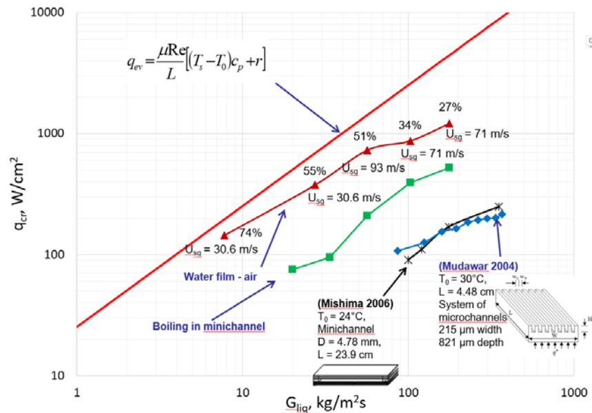
Рис. 53. Зависимость критического теплового потока от расхода жидкости, [110].
