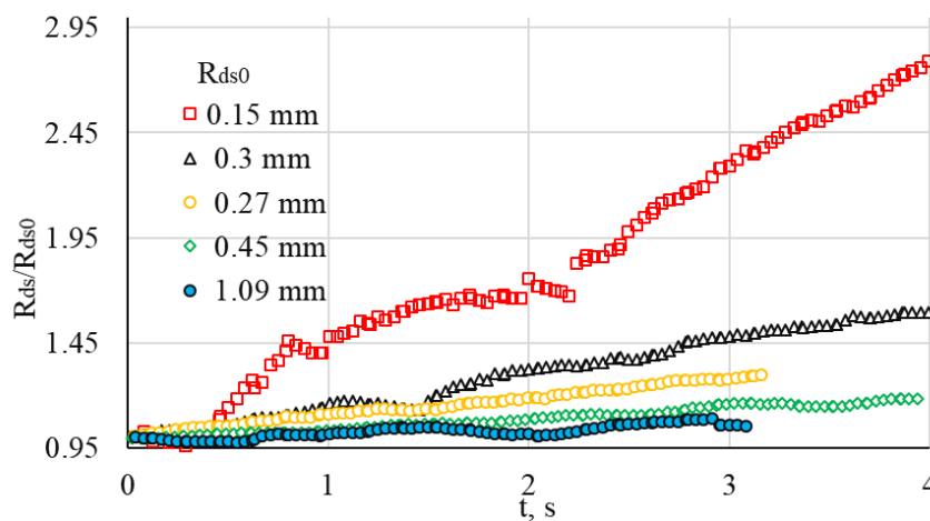
Рис. 8. Динамика контактной линии при мощности нагрева 1,22 Вт [4].
