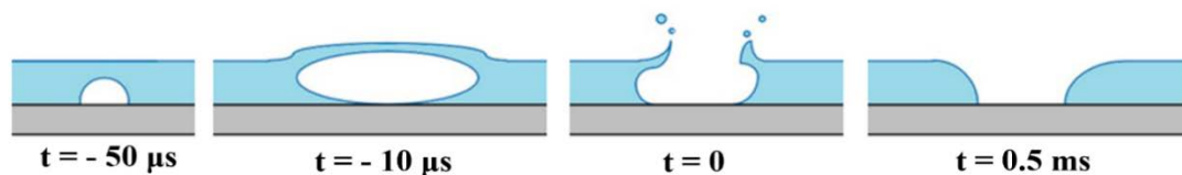
Рис. 48. Временная диаграмма образования сухих пятен в тонкой пленке жидкости.
