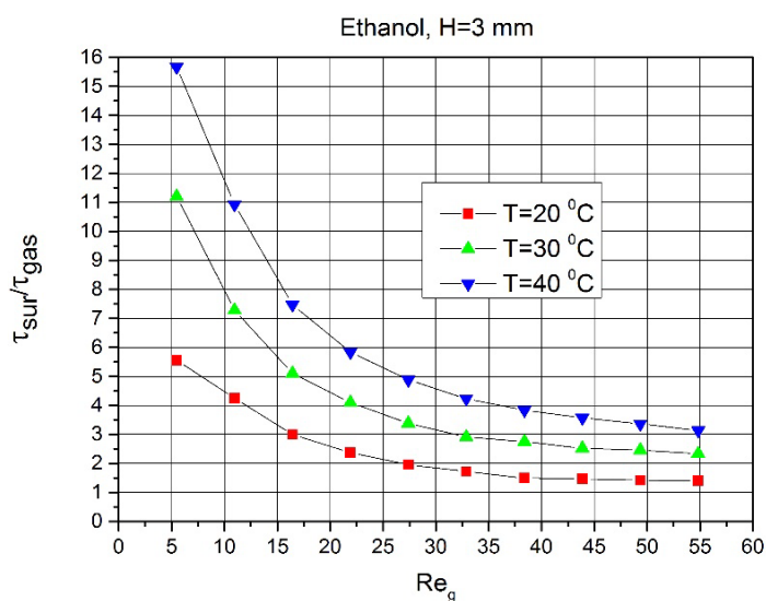
Рис. 9. Соотношение термокапиллярного касательного напряжения и касательного напряжения вызванного потоком газа (воздух) в зависимости от числа Re_g , [23, 52].
