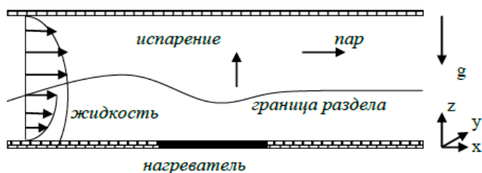
Рис. 3. Схема движения пленки жидкости в миниканале, [29].
