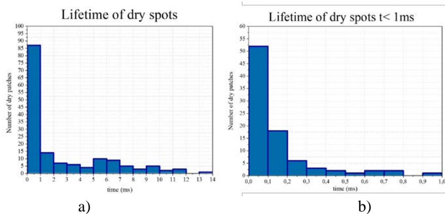
Рис. 51. Гистограмма срока жизни сухих пятен.
