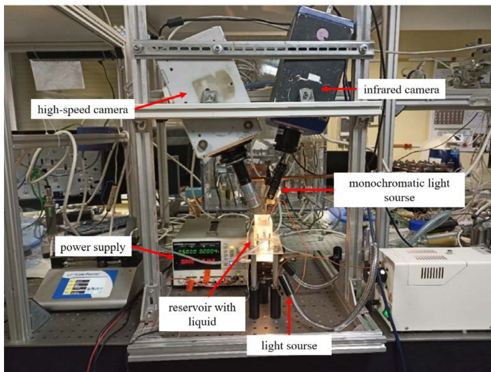
Рис. 5. Фото экспериментального стенда в ходе выполнения проекта РФФИ (2022 год).
