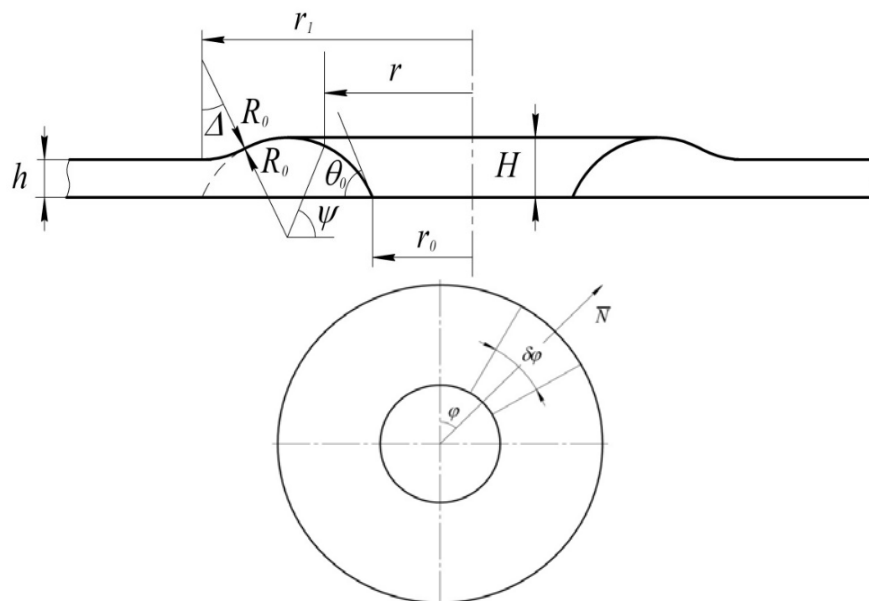
Рис. 25. Схематическое изображение сухого пятна в пленке жидкости, [21].
