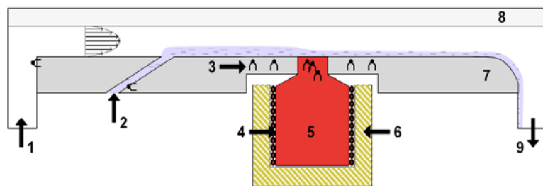
Рис. 45. Схема рабочего участка. 1 – вход газа; 2 – вход жидкости; 3 – термопары; 4 – нихромовая катушка; 5 – медный блок; 6 – теплоизоляция; 7 – стальная пластина; 8 – стеклянная пластина; 9 – выход жидкости и газа, [103].
