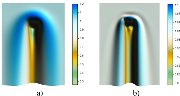
Рис. 4. Термокапиллярные деформации границы раздела газ-жидкость (вид сверху) с цветовыми шкалами деформаций, а) азот, б) водяной пар, размер нагревателя 3 x 6 мм, высота канала H_c=400 мкм, T_0= 30^\circ\text{C} , Re_l=5 , Re_g=8 , q=0.5 Вт/см 2 , [10].
