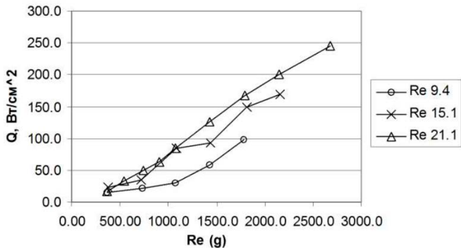
Рис. 29. Зависимость критического теплового потока от числа Рейнольдса газа для различных чисел Рейнольдса жидкости, [30,43].
