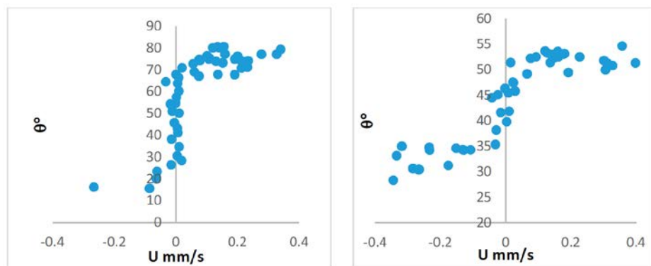
Рис. 17. Гистерезис контактного угла смачивания воды на сапфире (слева) и прозрачном нагревателе ИТО (справа), [12].
