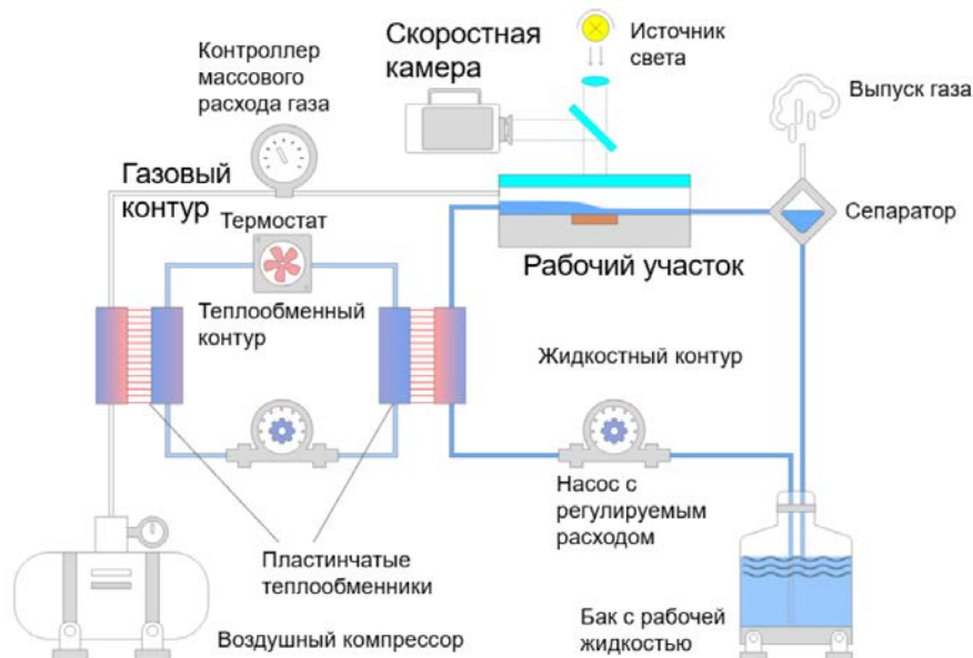
Рис. 1. Схема стенда, в котором для охлаждения локального источника тепла используется испарение тонкой пленки жидкости, увлекаемой потоком газа в канале (жидкостный контур замкнут, газовый контур разомкнут).
