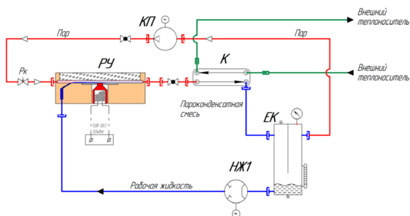
Рис. 38. Экспериментальный образец испарительной системы охлаждения теплонапряженных элементов с паровым компрессором. РУ – рабочий участок; НЖ1 – насос для жидкости; КП – компрессор паровой; К – конденсатор; ЕК – емкость конденсата; Рк – регулирующий клапан пара, [33].
