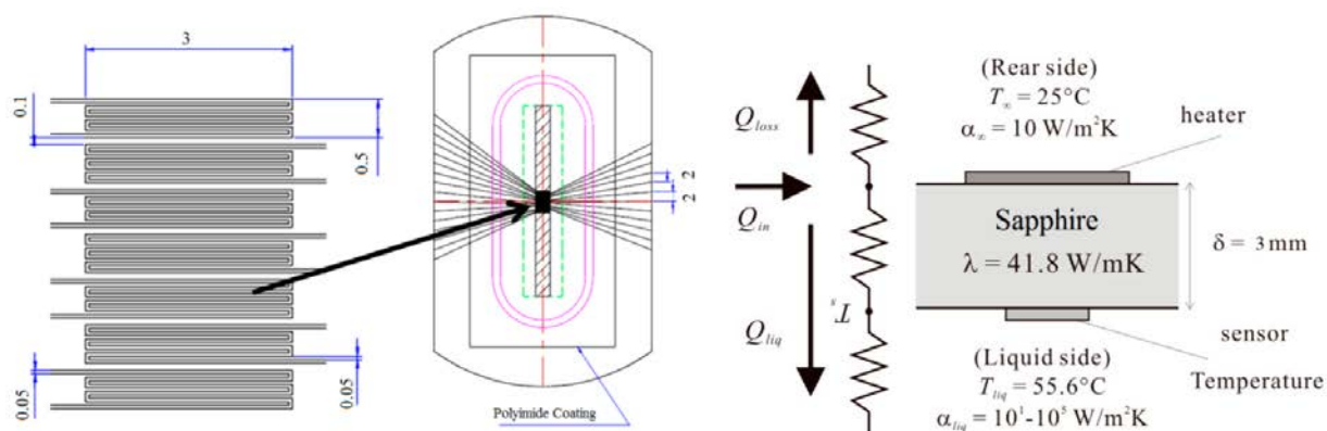
Рис. 14. Некоторые детали конструкции нагревательного элемента, изготовленного иностранным партнером, [12,30].
