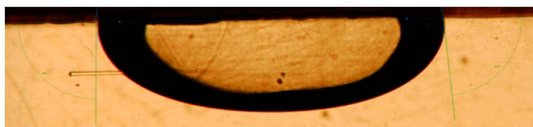
Рис. 19. Фотография пузырька в воде на прозрачном нагревателе ИТО, полученная теньевым методом, [31].
