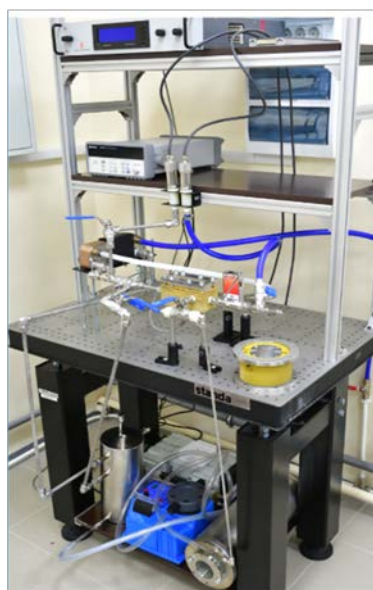
Рис. 37. Фотография экспериментального образца испарительной системы охлаждения теплонапряженных элементов с использованием однокомпонентных двухфазных потоков, [33].
