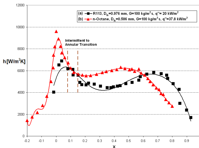
Рис. 1. Зависимость коэффициента теплоотдачи от паросодержания при кипении в миниканалах, «М-образный» закон: а) [76]; б) [77] (взято из [68]).
