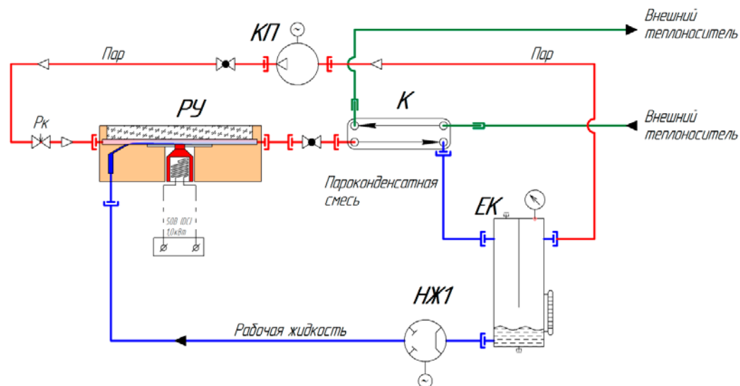
Рис. 5. Экспериментальный образец испарительной системы охлаждения теплонапряженных элементов с паровым компрессором. РУ – рабочий участок; НЖ1 – насос для жидкости; КП – компрессор паровой; К – конденсатор; ЕК – емкость конденсата; Рк – регулирующий клапан пара.
