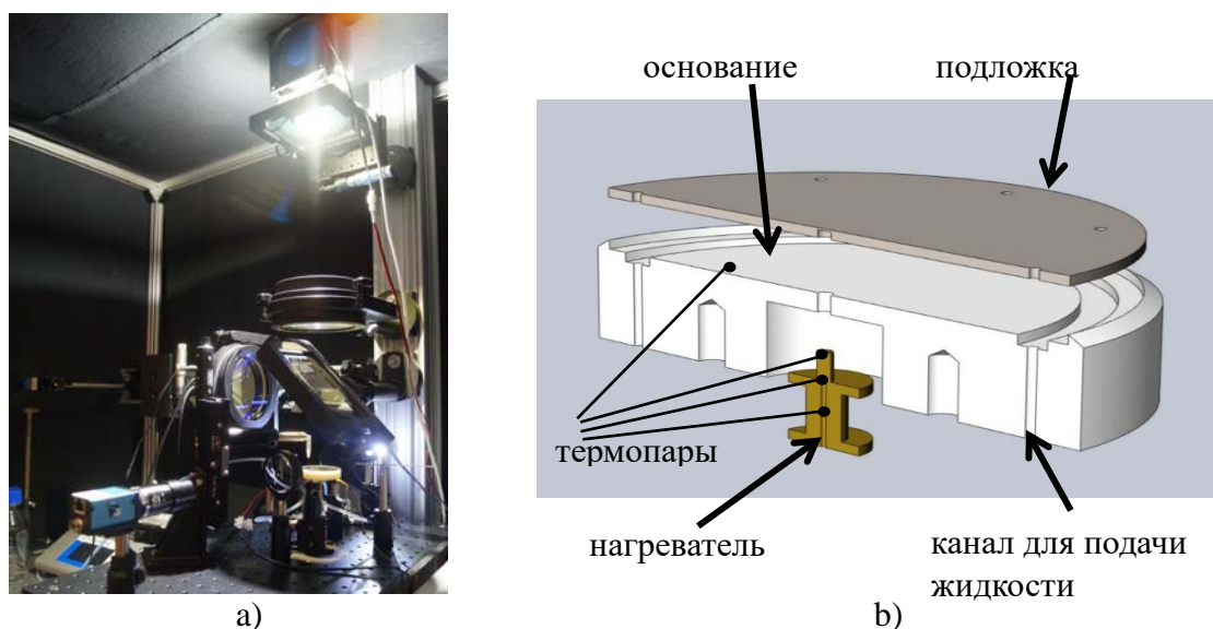
Рис. 23. Стенд для исследования разрыва горизонтального слоя жидкости с точечным нагревом: а) фотография штирен системы и рабочего участка; б) конструкция поверхности нагрева, диаметр подложки – 50 мм, толщина подложки – 1 мм, материал подложки – нержавеющая сталь, диаметр нагревателя – 1,6 мм, материал нагревателя – латунь, [51,43,48].
