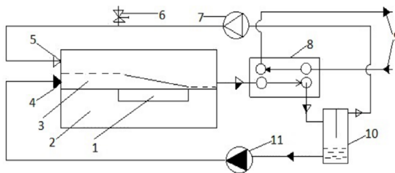
Рис. 4. Концепция системы охлаждения электронного оборудования с использованием чистого пара и парогазовой смеси: 1 –электронный компонент; 2 – подложка; 3 – испаряющаяся плёнка жидкости; 4 – вход жидкости в канал; 5 – вход парогазовой смеси в канал; 6 – клапан для сброса и регулировки концентрации неконденсируемого газа; 7 – компрессор; 8 – пластинчатый теплообменник (конденсатор пара); 9 – система охлаждения конденсатора; 10 – сепаратор, совмещенный с баком-накопителем для жидкости и газовой фазы; 11- жидкостный насос.
