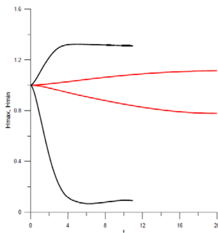
Рис. 6. Безразмерная максимальная и минимальная толщина пленки в зависимости от безразмерного времени (реальное время развития процесса 4 с, обезразмеривание выполнено делением на начальную толщину пленки): черная линия - газ азот; красная линия - водяной пар, размер нагревателя 3 x 6 мм, высота канала H_C=300 мкм, T_0=30^\circ\text{C} , Re_l=2.5 , Re_g=4 , q=0.5 Вт/см 2 , [30].
