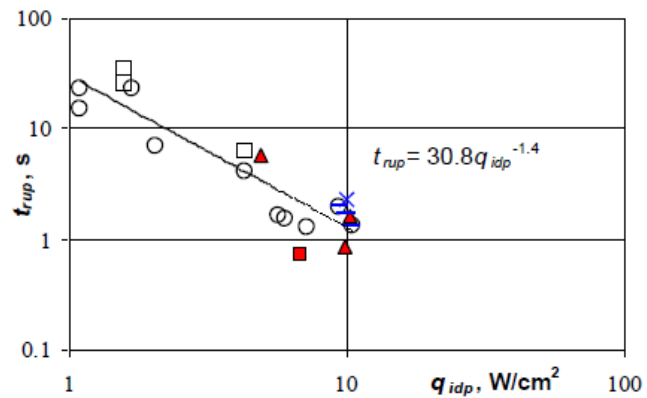
Рис. 18. Время образования сухого пятна в зависимости от плотности теплового потока, [31].
