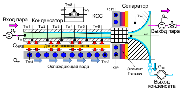
Рис. 33. Схема конденсационно - сепарационной системы, [32].
