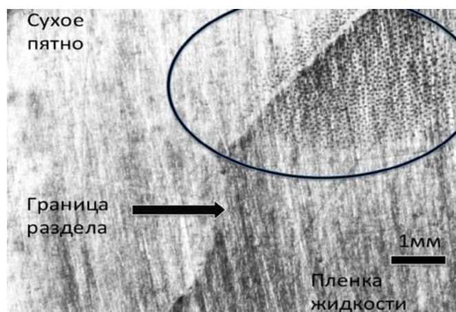
Рис. 22. Локально нагреваемый горизонтальный слой воды: нагреватель 1 \times 1 см 2 , толщина слоя 0.4 мм, тепловой поток 27.5 Вт/см 2 , область монослоя из микрокапель конденсата обведена овалом, в области линии контакта газ – жидкость – твердое тело микрокапли не могут существовать (белая полоска внутри овала), по-видимому, микрокапли ее перепрыгивают, [37].
