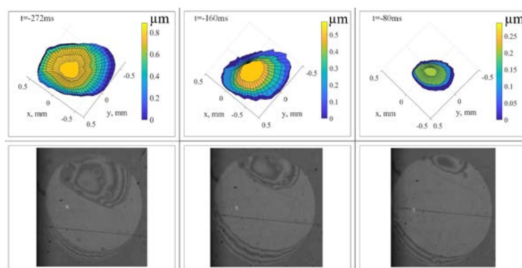
Рис. 7. Восстановленный профиль микрослоя, образовавшегося при слиянии двух пузырьков (вверху), интерференционные изображения (внизу) [4].
