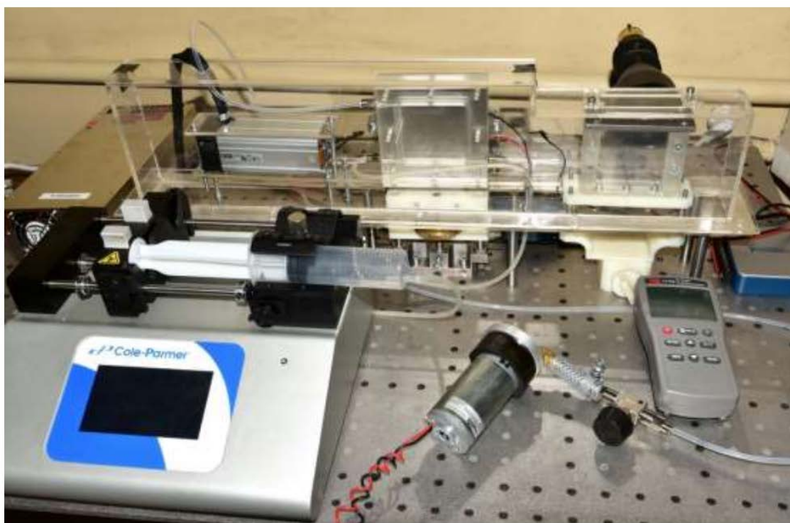
Рис. 3. Фото стенда, приведенное в отчете проекта ФЦП № 14.613.21.0011, соглашение от 27.08.2014 г.
