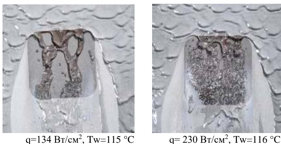
Рис.30. Разрушение пленки воды при локальном нагреве в плоском горизонтальном миниканале при Re_l = 21,1 и Re_g = 2700 . Течение направлено сверху вниз, [31].
