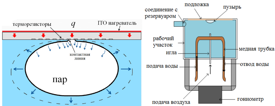
Рис. 4. Концепция стенда.
