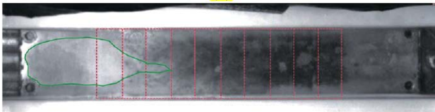
Рис. 43. Формирование крупных сухих пятен в пленке жидкости, вода, Re_1=42 , Re_g=2540 , T_{1in}=40\text{ }^\circ\text{C} , q=20\text{ Вт/см}^2 .
