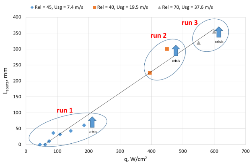
Рис. 52. Общая длина линии контакта на нагревателе размером 10x10 мм 2 в зависимости от теплового потока (вода).
