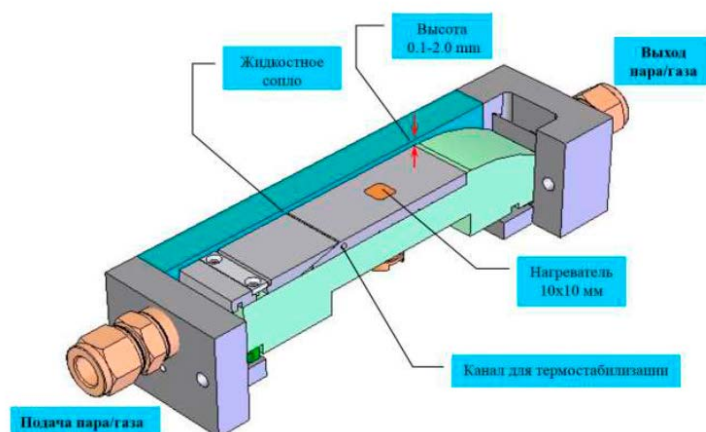
Рис. 27. Стенд для экспериментального исследования гидродинамики, теплообмена и кризисных явлений в пленке жидкости, движущейся под действием потока газовой фазы, [30,43].
