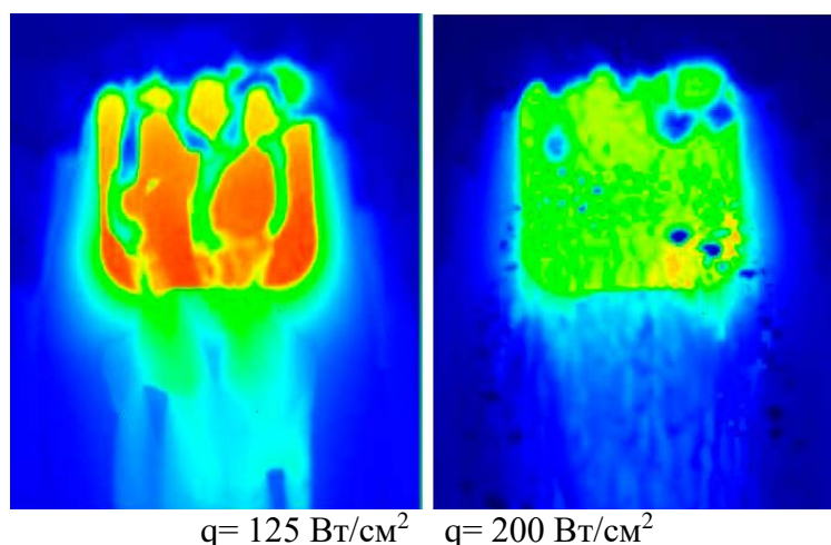
Рис. 31. Разрушение пленки воды при локальном нагреве в плоском горизонтальном миниканале при Re_l = 30 и Re_g = 2200 . Течение направлено сверху вниз, [30].
