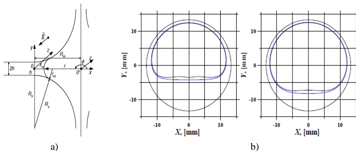
Рис. 34. Моделирование положения мениска в сепараторе: а) схема мениска; б) сравнение эксперимента (черная линия) и расчета (синяя линия), [32].
