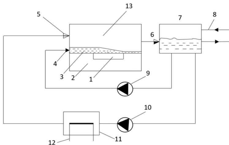
Рис. 3. Концепция системы охлаждения электронного оборудования с использованием чистого пара: 1 –электронный компонент; 2 – подложка; 3 –испаряющаяся плёнка жидкости; 4 – вход жидкости в канал; 5 – вход пара в канал; 6 – вход жидкости и пара в конденсатор; 7 – конденсатор пара и резервуар для жидкости; 8 – система охлаждения конденсатора; 9 –насос для подачи жидкости в канал; 10 – насос для подачи жидкости в парогенератор; 11- парогенератор и резервуар для пара; 12- электрический подогреватель; 13 – мини или микро-канал.
