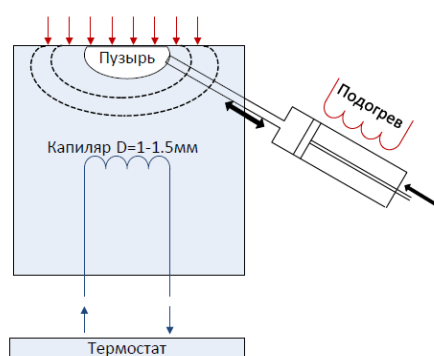
Рис. 11. Концепция стенда: создание линии контакта посредством пузырька газа или пара под нагреваемой прозрачной поверхностью, [29,45].
