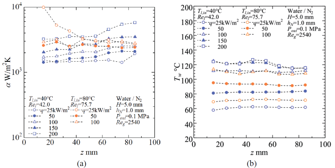
Рис. 42. Локальный коэффициент теплопередачи и распределение температуры поверхности вдоль потока при различных сочетаниях теплового потока и температуры жидкости на входе, [6,31].
