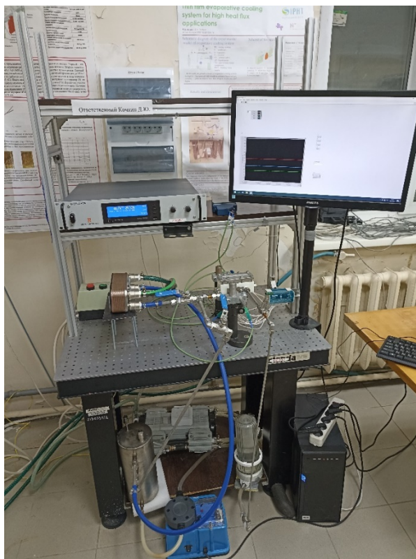
Рис. 2. Фото экспериментального стенда, воссозданного в соответствии с приказом директора ИТ СО РАН, март 2024 года.
