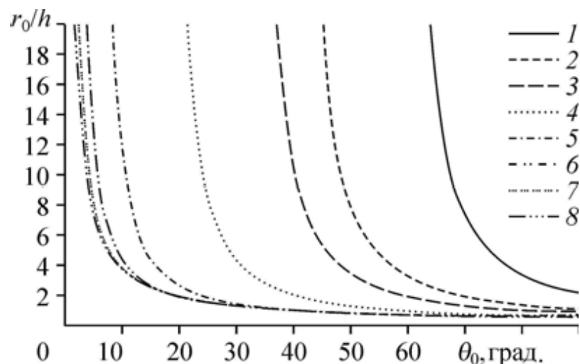
Рис. 26. Результаты расчетов критических значений радиуса сухого пятна в пленке жидкости в зависимости от равновесного краевого угла смачивания и числа Бонда. Bo = 1 (1), 2 (2), 3 (3), 10 (4), 10^{-2} (5), 10^{-3} (6), 10^{-4} (7), 10^{-6} (8), [22].
