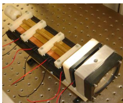
Рис. 32. Стенд для исследования процессов в пассивной конденсационно-сепарационной системе, [32].
