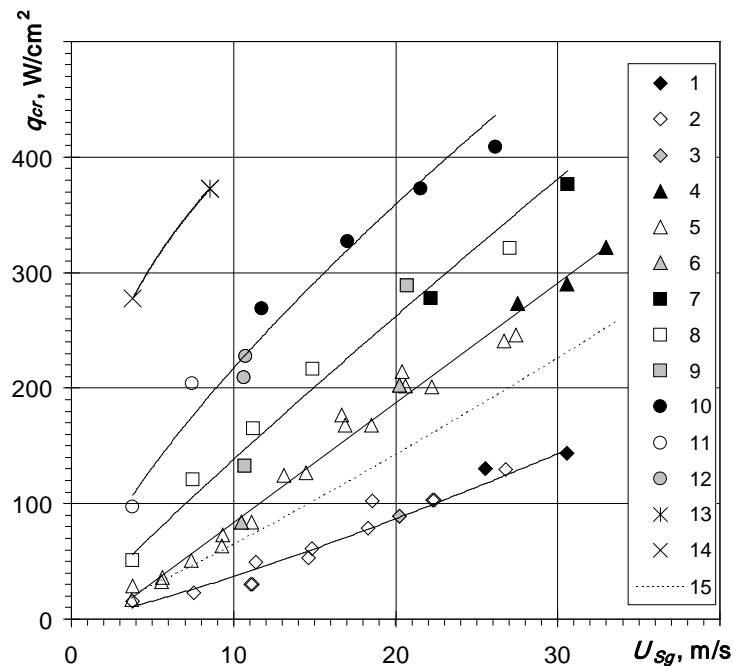
Рис. 2. Критический тепловой поток, в зависимости от приведенной скорости газа в канале U_{sg} , для различных чисел Рейнольдса жидкости Rel и различных высот канала H : 1- Rel=8.5 , H=1.2 mm; 2- Rel=8.5 , H=1.5 mm; 3- Rel=8.5 , H=2 mm; 4- Rel=20 , H=1.2 mm; 5- Rel=20 , H=1.5 mm; 6- Rel=20 , H=2 mm; 7- Rel=30 , H=1.2 mm; 8- Rel=30 , H=1.5 mm; 9- Rel=30 , H=2 mm; 10- Rel=46 , H=1.2 mm; 11- Rel=46 , H=1.5 mm; 12- Rel=46 , H=2 mm; 13- Rel=84 , H=1.2 mm; 14- Rel=84 , H=1.5 mm; 15- обобщение данных для Rel=14 , H=1.2-2 mm [2].
