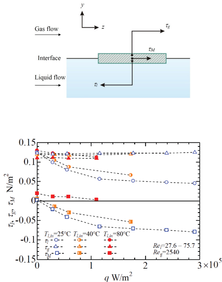
Рис. 44. Упрощенный баланс сил в пленке жидкости и карта сдвиговых напряжений в пленке жидкости, [8,31].
