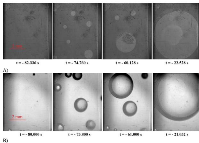
Рис. 6. Последовательность изображений динамики парогазовых пузырьков под прозрачной нагреваемой подложкой [4].
